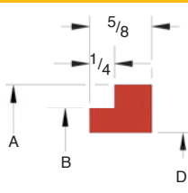
L-Shape
